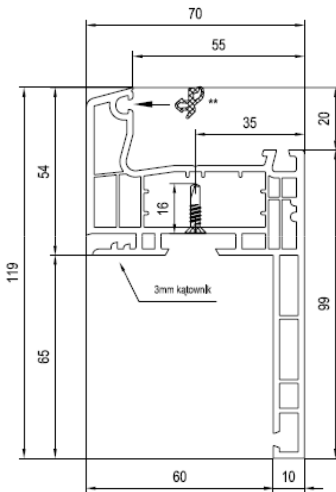
640311 Mostek szklenia zintegrowany z 5mm podkładką
